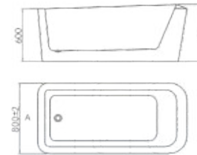
Size:1800×900×600mm 1700×800×600mm
