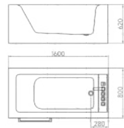
Size:1600*800*620mm
