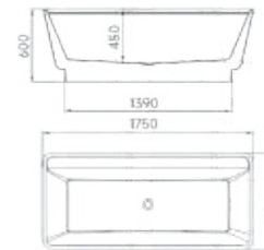
Size:1750×800×600 mm
